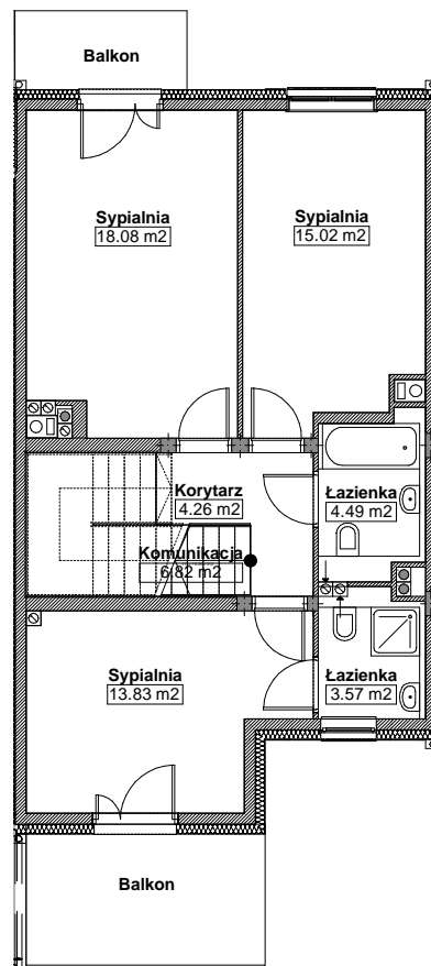
1 RZUT_PIĘTRA
