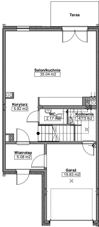
0 RZUT_PARTERU
