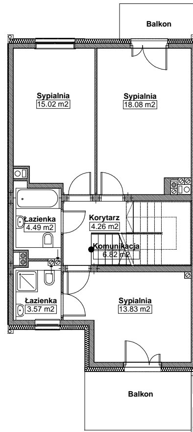
1 RZUT_PIĘTRA
